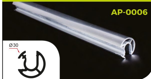
PROFIL Ø30 SA 2 KANALA - 6 met.
