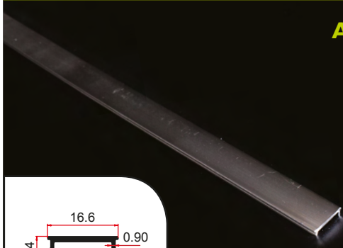
MASKA PROFILA AP-24A
