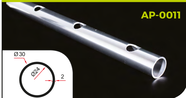
PROFIL Ø30 BUŠENI - 3 met.
